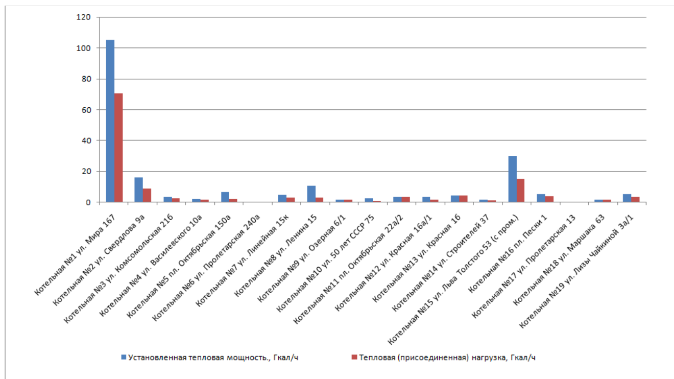
Диаграмма 2.1 Баланс тепловой мощности
